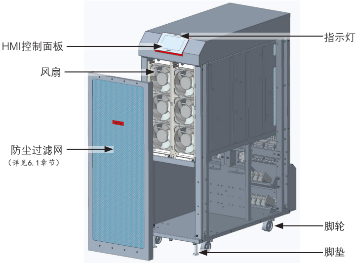
60K/80K 机柜结构图：
