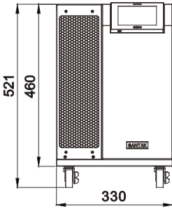
前视图
